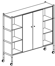
Struttura per lavagna / monitor Structure for white board / screen 209 x 53 x 177h. cm
