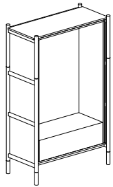
Seduta singola - Single seat 108 x 53 x 177h. cm
