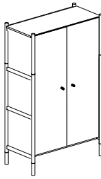
108 / 158 x 53 x 177h. cm
