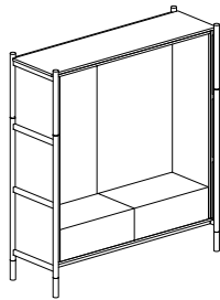
Seduta doppia - Double seat 158 x 53 x 177h. cm
