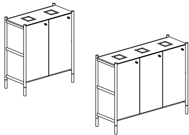
108 / 158 x 53 x 127h. cm
